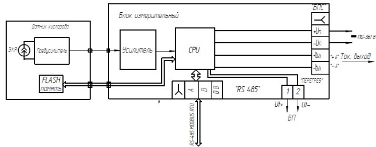
Рисунок 16 – Анализатор АНКАТ 7655-03. Схема функциональная
