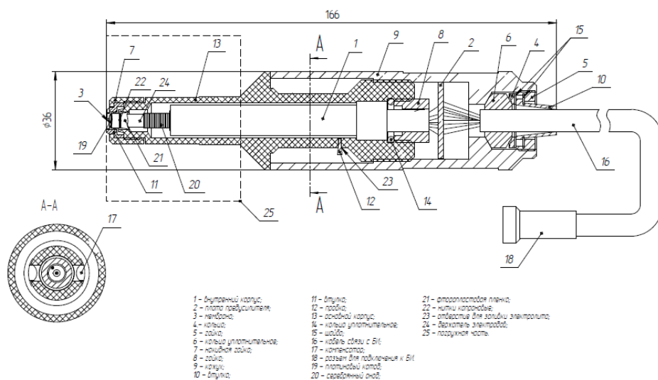
Рисунок 13 – Внешний вид и конструкция датчика
