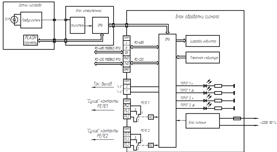
Рисунок 15 – Анализатор АНКАТ 7655-02. Схема функциональная
