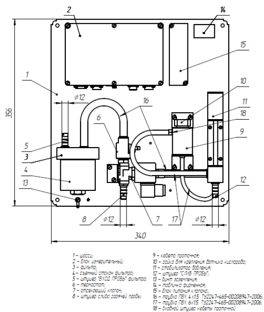
Рисунок 14 – Внешний вид РЭ
