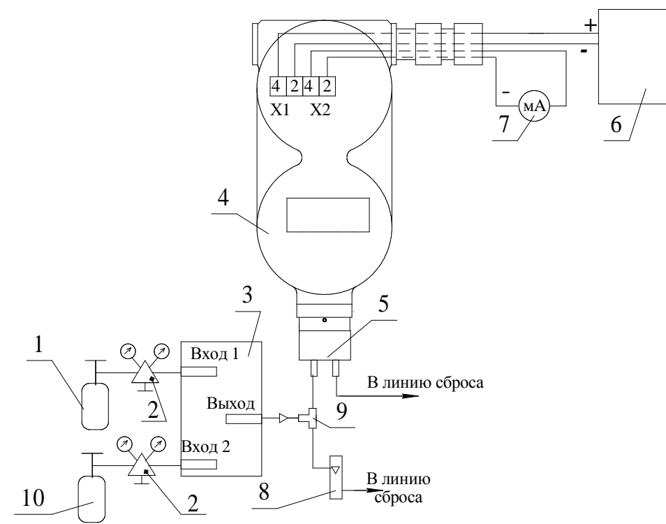
б) для газоанализаторов ДАФ-М-05Х/-08Х/-06ТРХ/-08ТРХ
