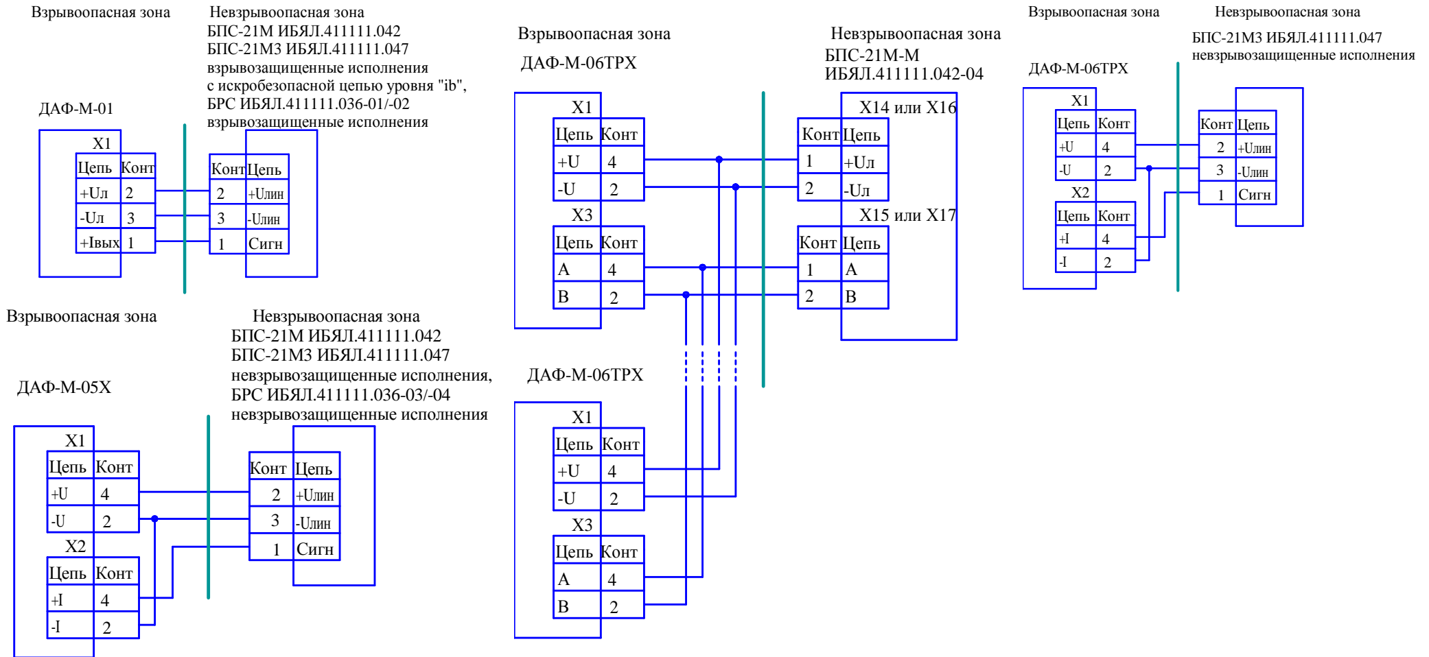
Рисунок П.1 - Схема подключения газоанализаторов ДАФ-М к блокам БПС-21МЗ, БПС-21М, БРС
