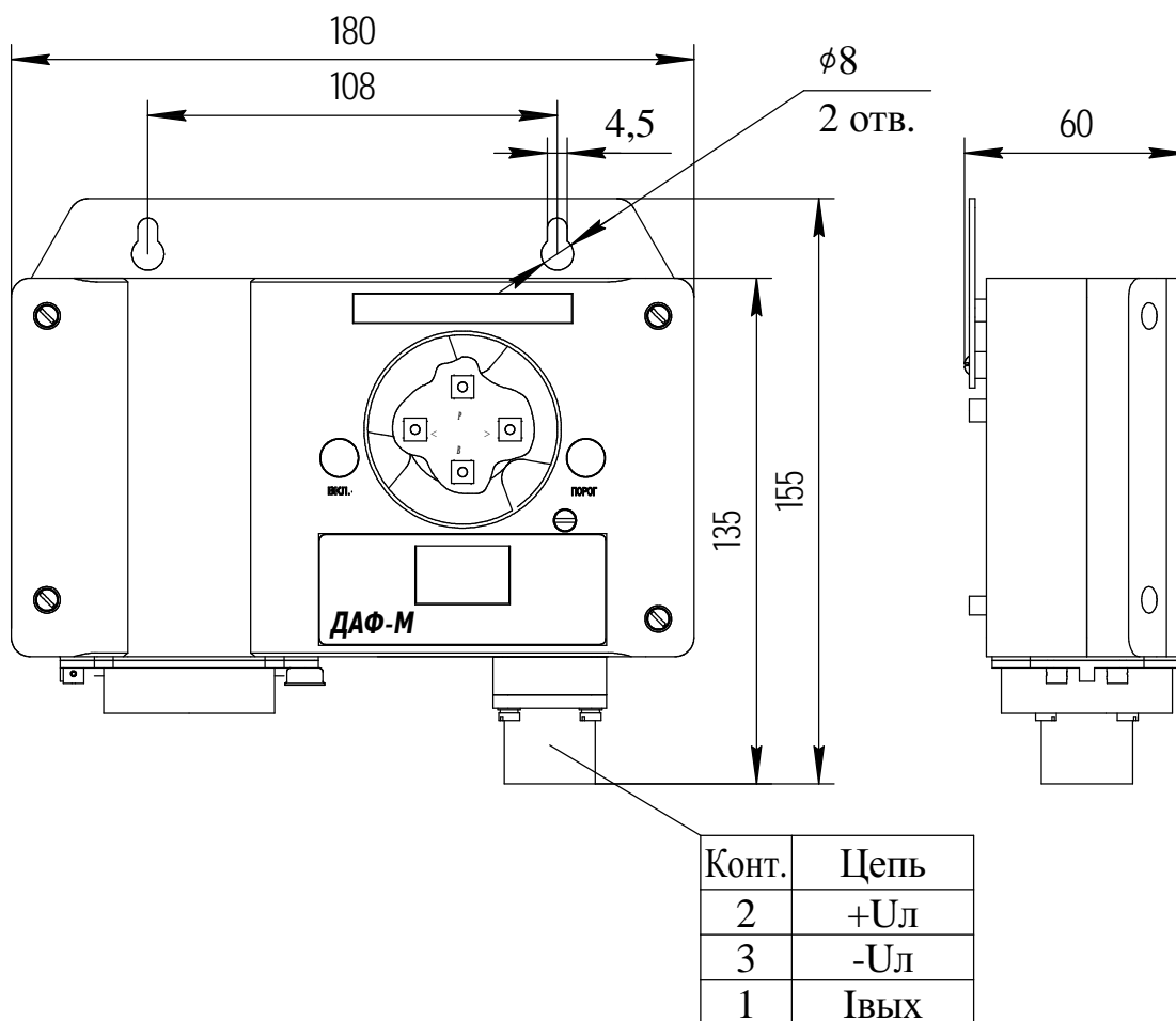
Рисунок Л.1 - Монтажный чертеж газоанализаторов ДАФ-М-01
