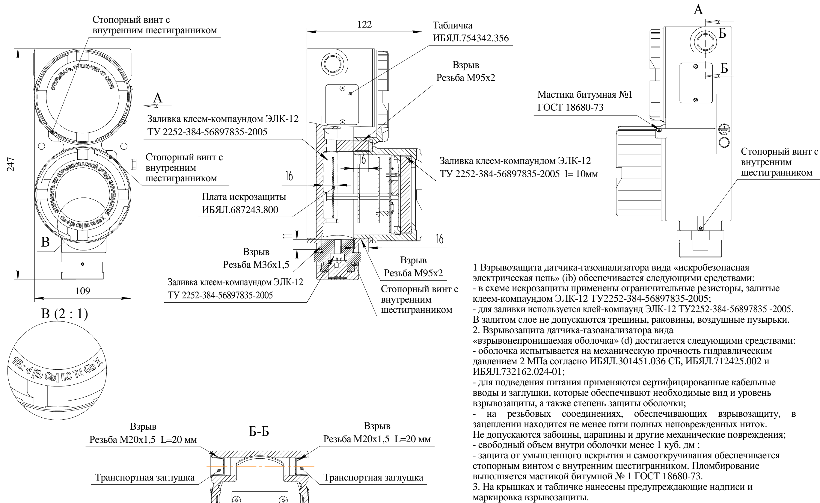
Рисунок Е.2 - Чертеж средств взрывозащиты датчиков-газоанализаторов ИБЯЛ.413445.003-06 (-09)
