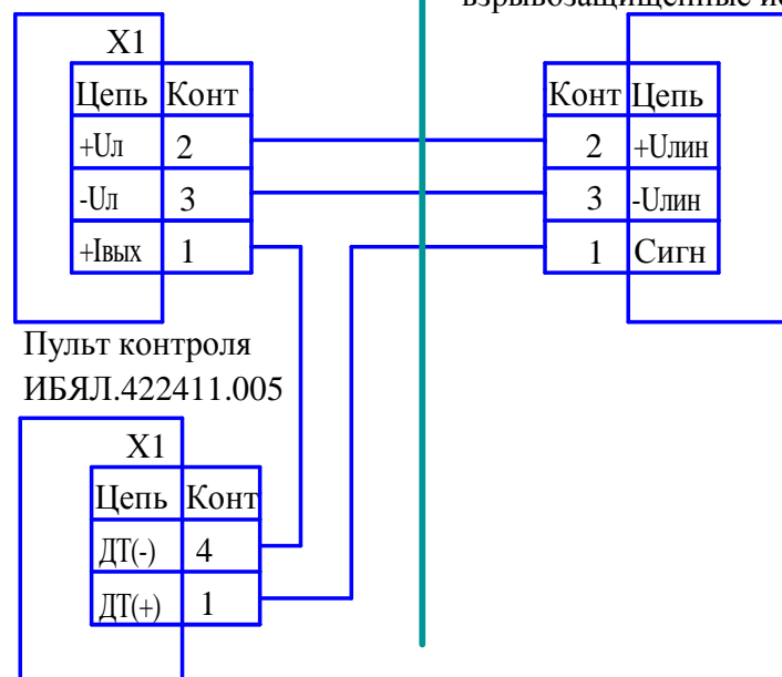
Рисунок П.2 - Схема подключения
