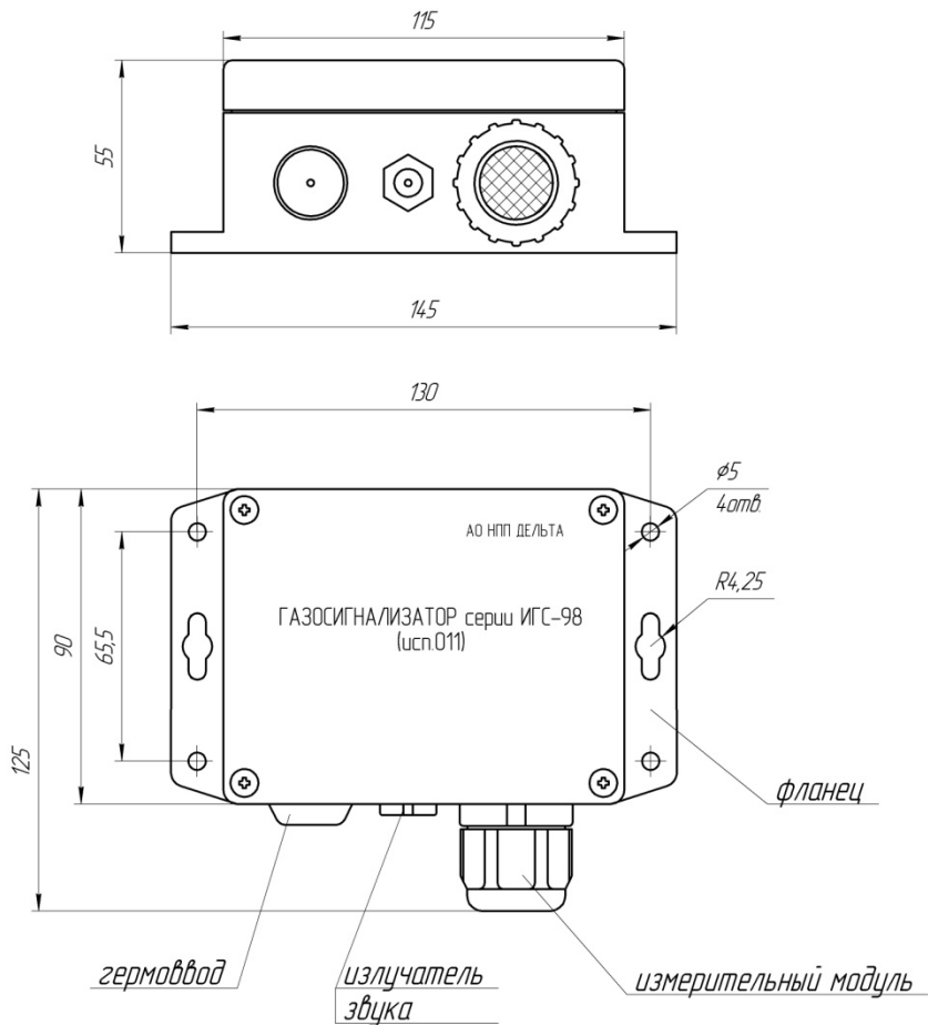
Рис.1 Габаритный чертеж газосигнализатора
