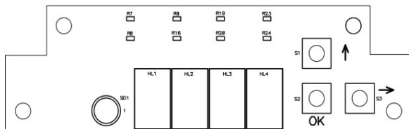
Рис. 4 Чертеж платы индикации и управления
