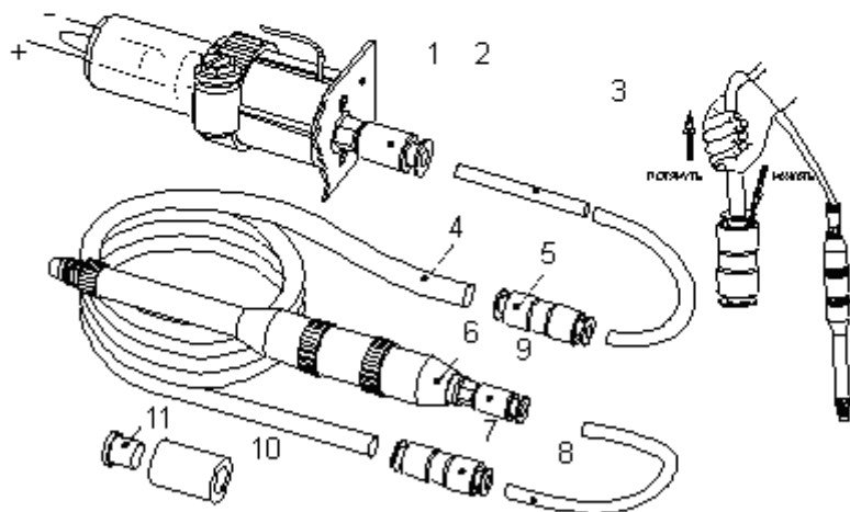
Рис. 4. Схема соединения элементов удлинителя с газоанализатором
