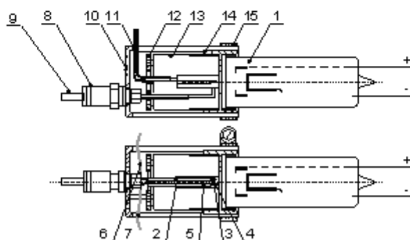
Рис. 2. Фотоионизационный детектор.
