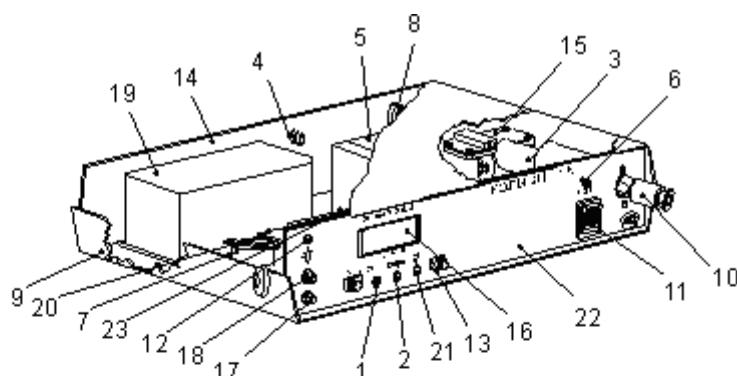
Рис. 1. Газоанализатор КОПИОН - 1 А.
