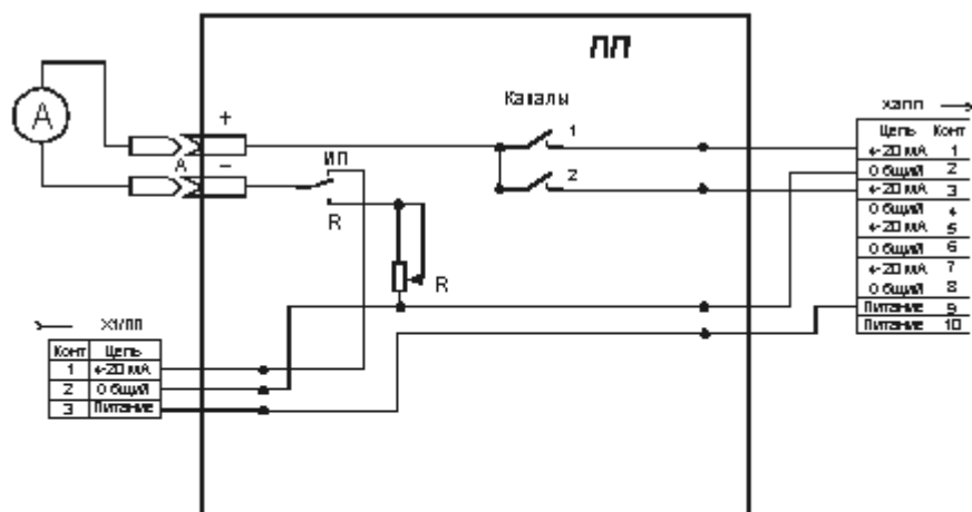
РИС. 6 Схема пульты поверочной для проверки работоспособности БМС, проверки работоспособности и градуировки газоанализаторов.
