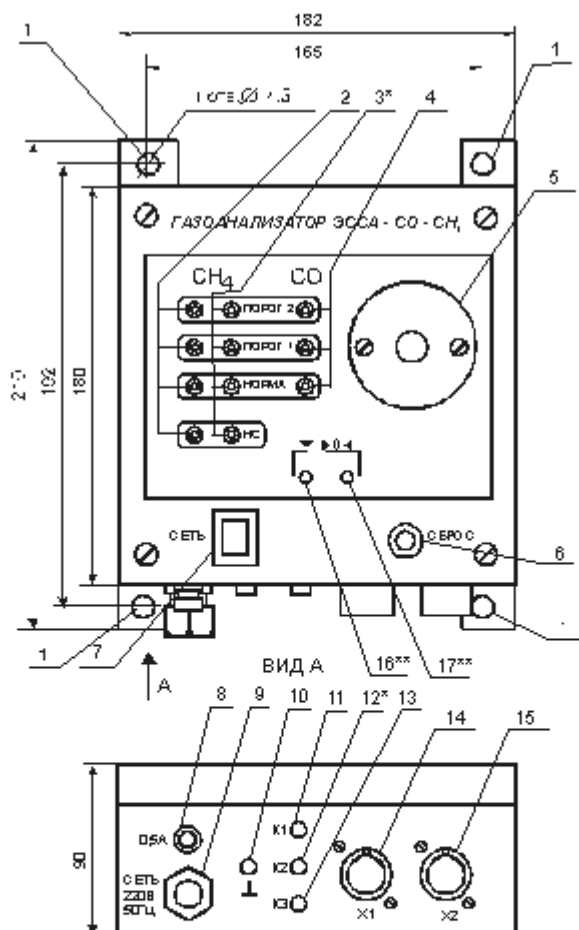
РИС 2. БИС газоанализаторов ЗССА - CO - CH 4 , ЗССА - CO - CH 4 /2 габаритные и установочные размеры.
