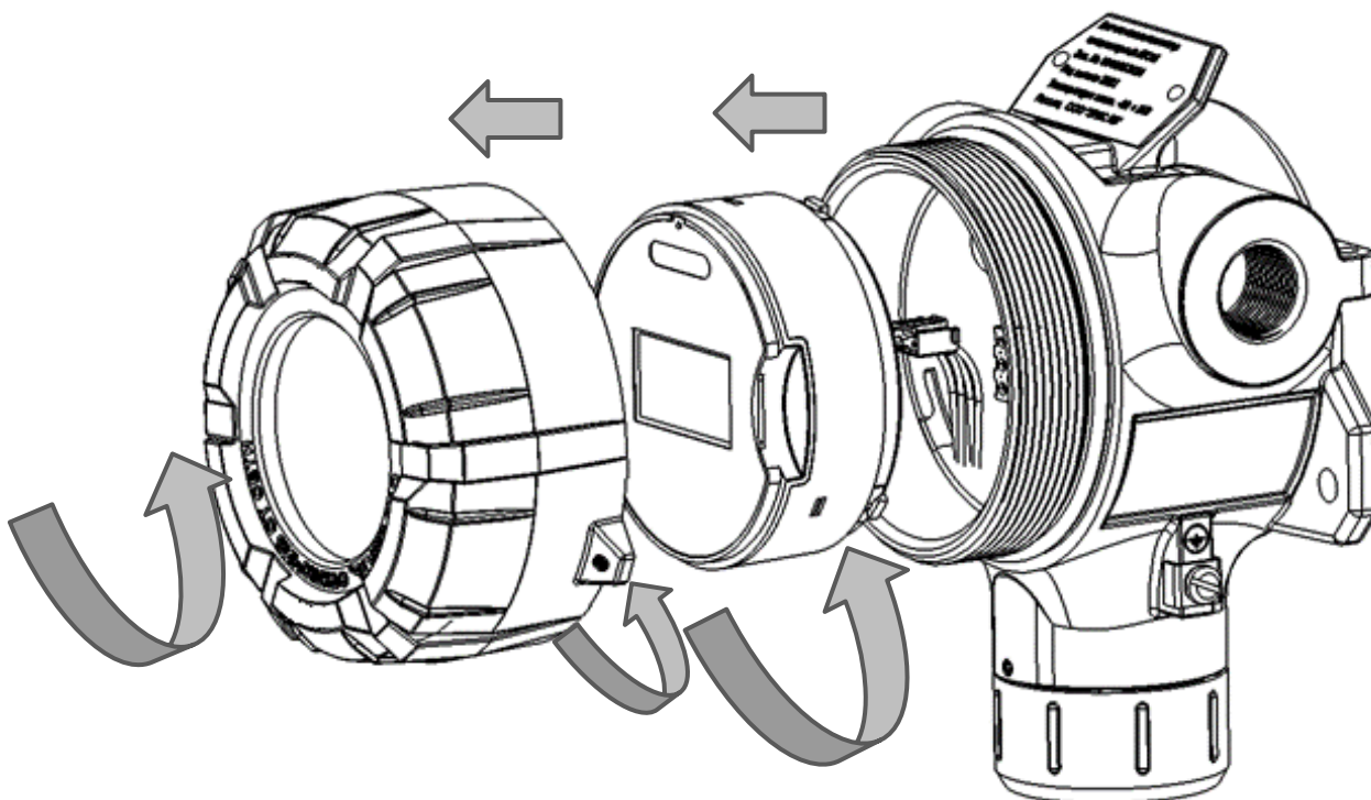
Рисунок 14- Схема разбора газоанализатора
