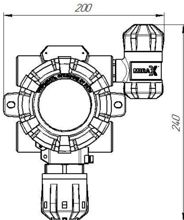
Рисунок 2 – Габаритные размеры AXIOM
