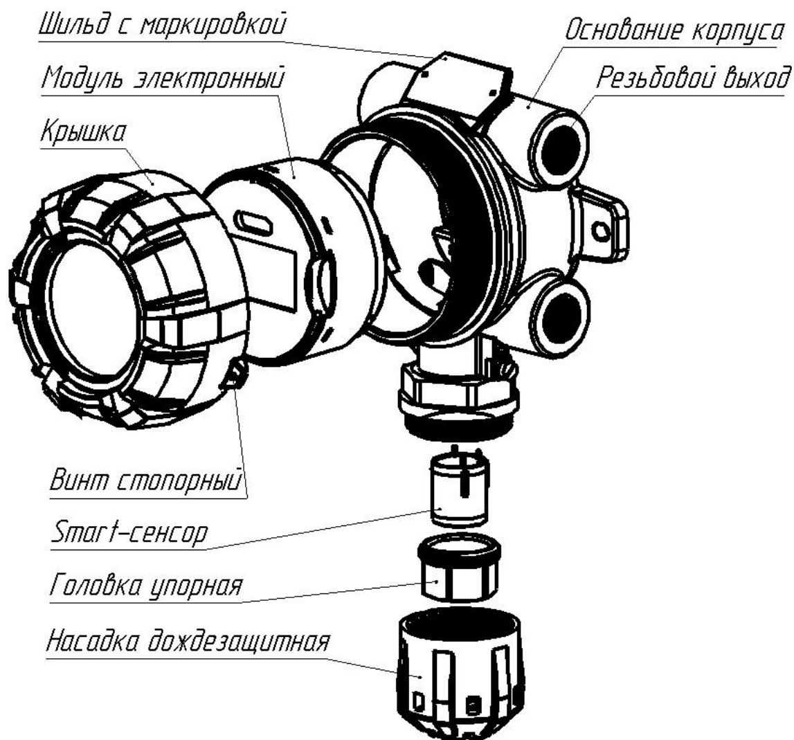
Рисунок 3 – Функциональный состав AXIOM
