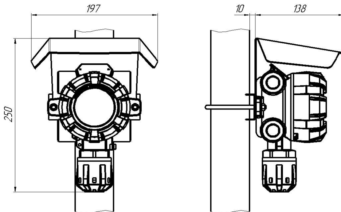
Рисунок 11 - Монтаж козырька газоанализатора
