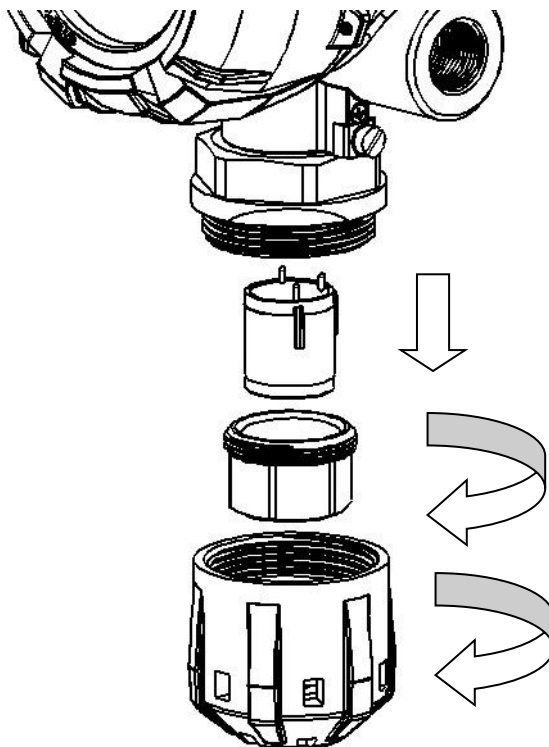
Рисунок 15 – Схема разборки при замене сенсора
