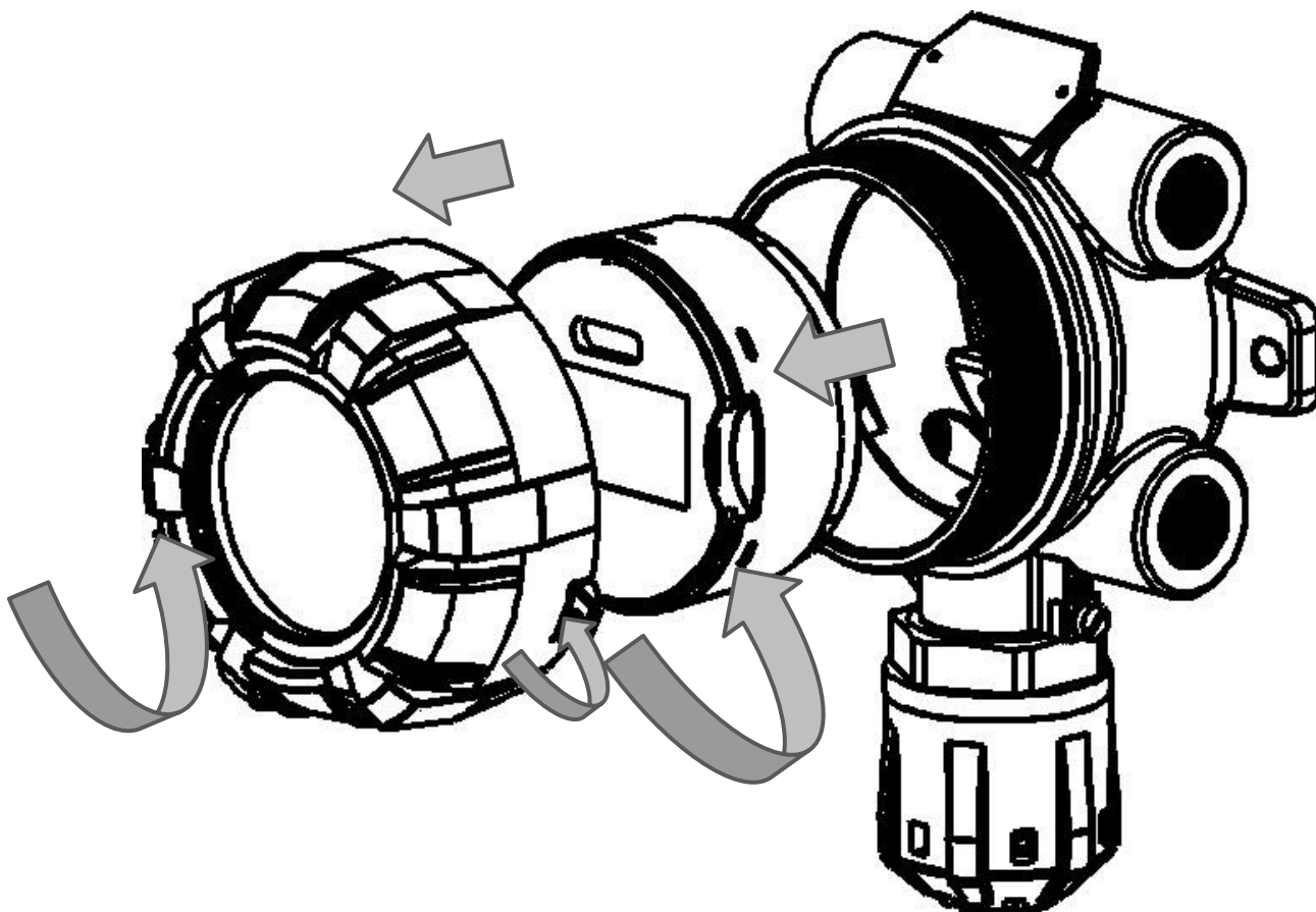
Рисунок 15 - Схема разбора газоанализатора
