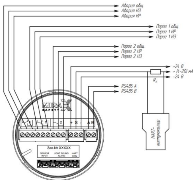
Рисунок 13 – Схема подключения газоанализатора AXIOM
