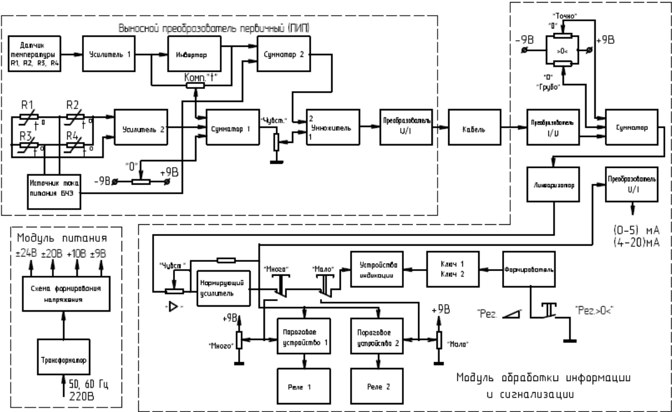
Рисунок 12 – Газоанализаторы ГТВ-1101 ВЗ-А. Схема электрическая структурная
