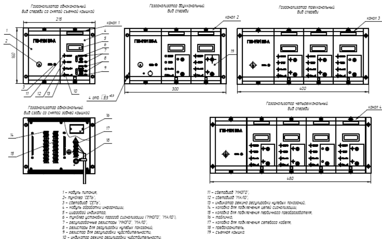
Рисунок 11 – Газоанализаторы GTB-1101 B3-A. Внешний вид
