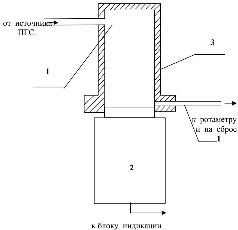
Рисунок 1 - Подача ПГС в адаптер при проверках 1 – соединительные трубки; 2 – блок датчиков; 3 – адаптер
