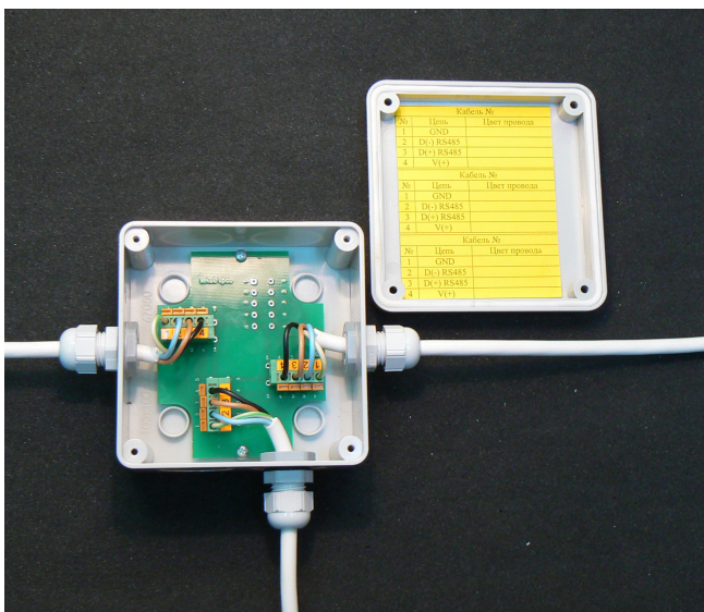
Рис.Д.10. Монтажный комплект МКУ со снятой крышкой
