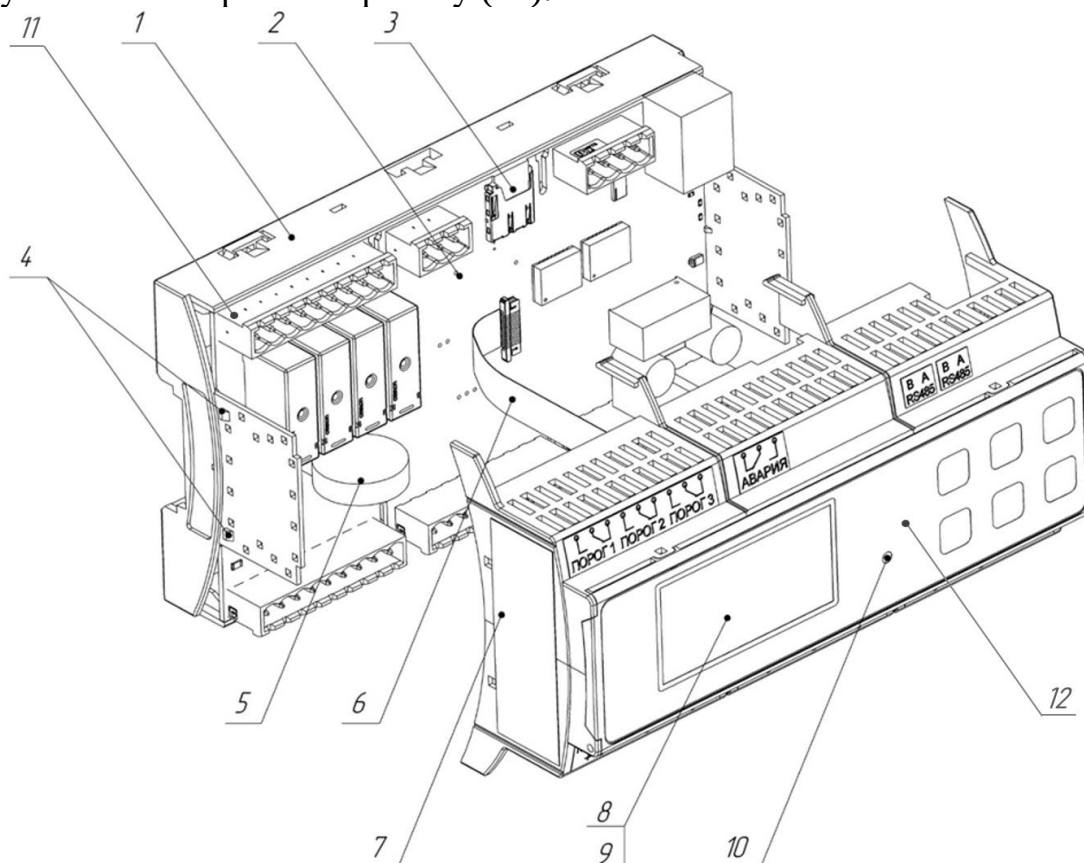
Рисунок 35 – Устройство контроллера
