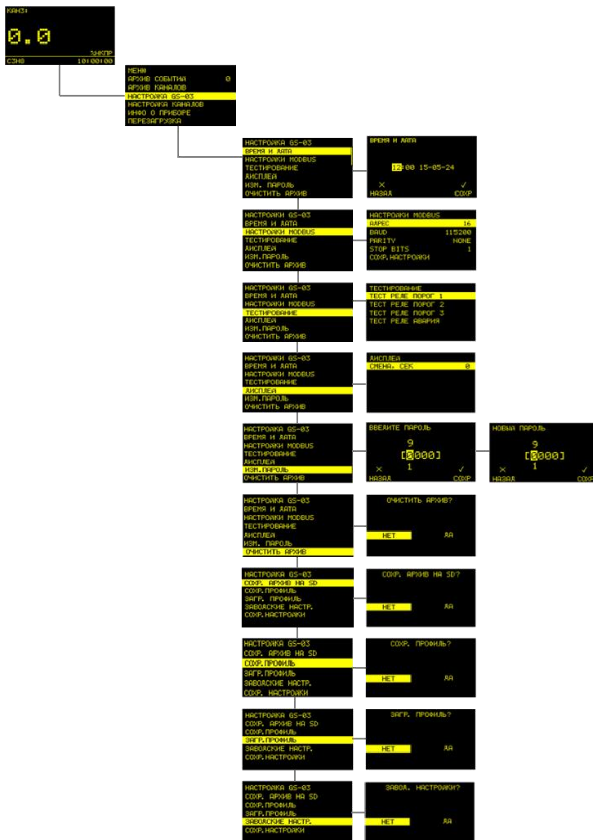
Рисунок Г.3 – Подменю «НАСТРОЙКА GS-03»
