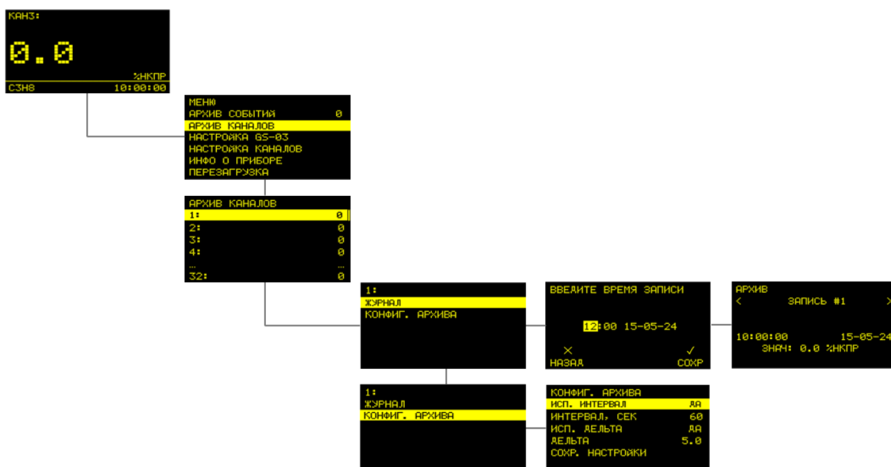
Рисунок Г.2 – Подменю «АРХИВ КАНАЛОВ»
