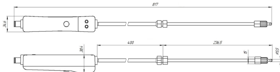
Рисунок А.2 – Габаритные размеры устройства с зондом 600 мм
