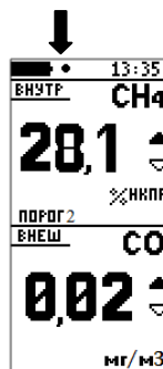
Рис. 10 Индикация режима автозаписи на экране Сигнализатора
