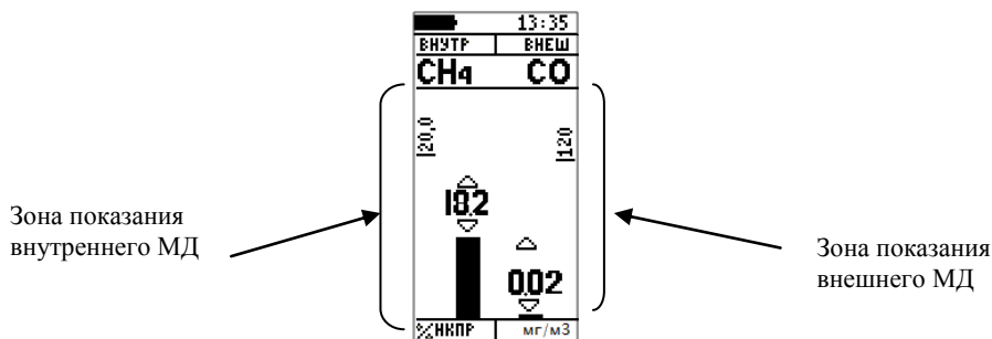
Рис.7.2 Режим измерения при графическом отображении индикатора (для датчиков на метан и оксид углерода)
